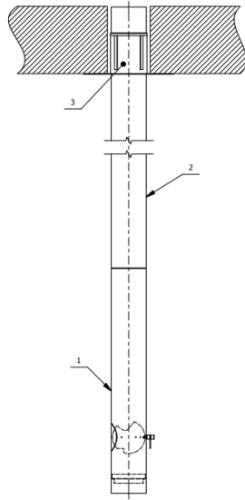
Schemat IV - Kominek (koza) wolnostojący (środek pomieszczenia) Przykład budowy przyłącza kominowego z płytą okrągłą z wkładką dwuścienną.
