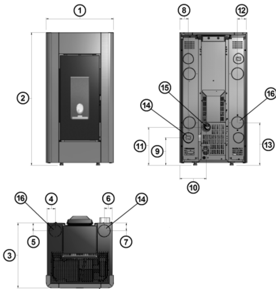
Fig. 19 - Ogólne wymiary: Prince 3 11KW / Prince 3 Plus 11KW
