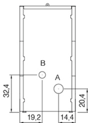
POSTERIORE - BACK - POSTERIEUR - HINTER
