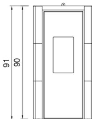
FRONTALE - FRONT - AVANT - VORDER
