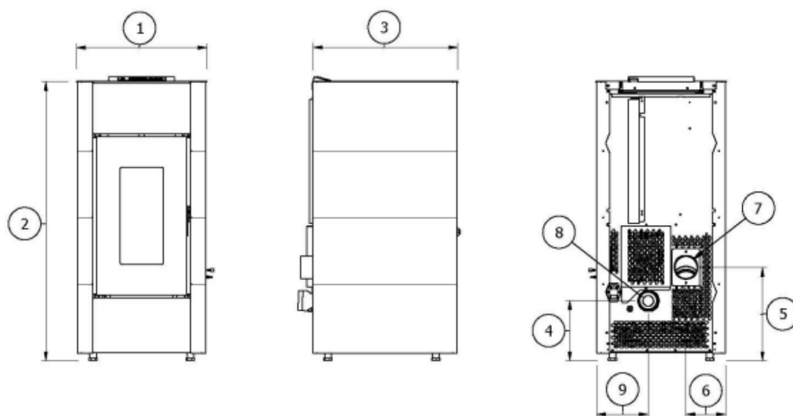
Fig. 24 - Ogólne wymiary: Cristal ®
