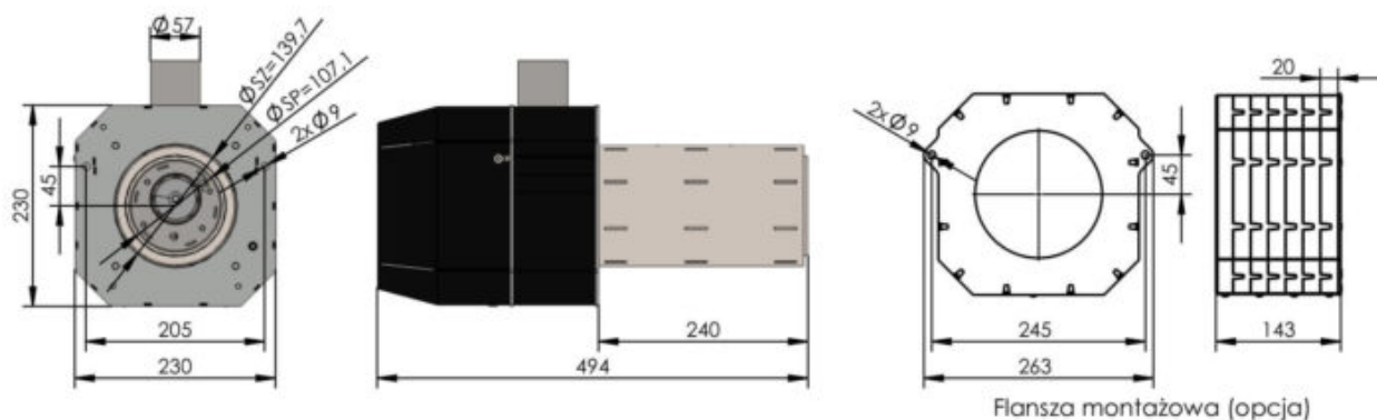
Rysunek palnik pelletowy 36 kW
