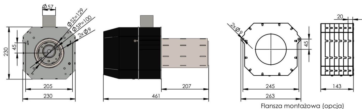
Rysunek palnik pelletowy 26 kW
