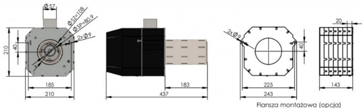
Rysunek palnik pelletowy 16 kW
