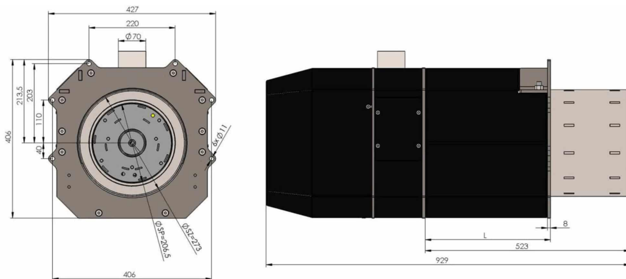
Rysunek palnik pelletowy 150 kW
