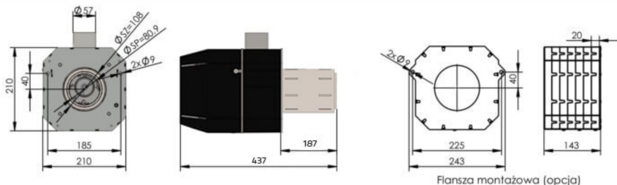
Rysunek palnik pelletowy 10 kW
