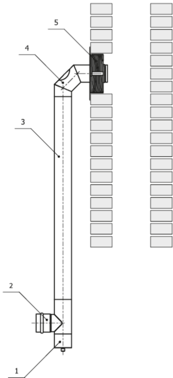
Rys. Przykład budowy przyłączaz elementów systemu SPP
