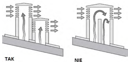
Rys. Charakterystyka komina
