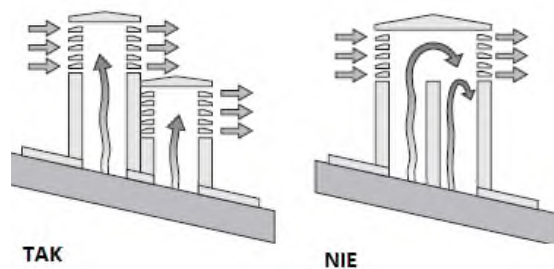
Rys. Charakterystyka kominy
