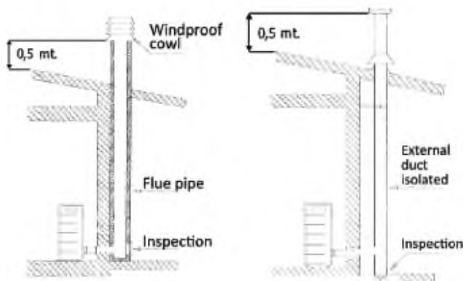
Rys. 2 podłączenie do przewodu spalinowego
